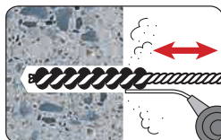
② 孔内清掃(2~3回繰返し)
